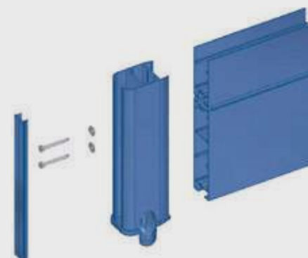
Dimensions du montant 90 x 60 mm
